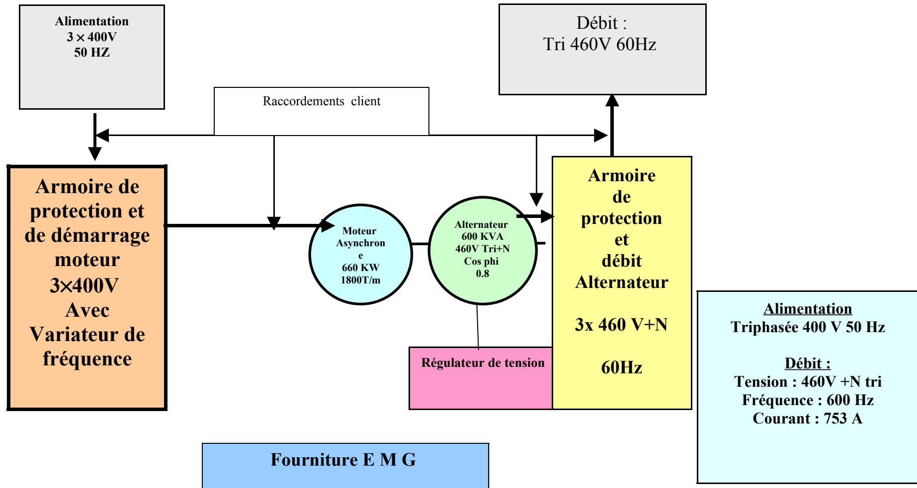
Schéma de principe
